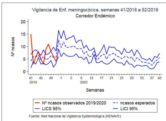
Corredor endémico para la temporada 2019/20
