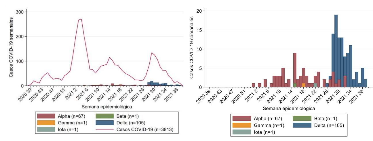
Figura 14. Detecciones de SARS-CoV-2 con información de caracterización genética por semana epidemiológica de toma de muestra. Sistema centinela. Temporada 2020-21. España.
